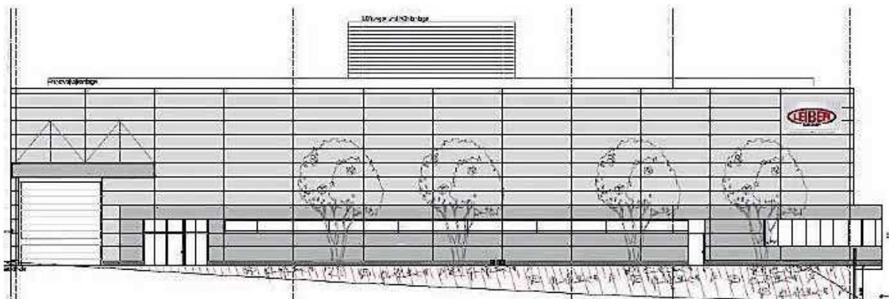
Westansicht der geplanten Produktionshalle
